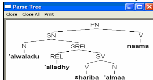
Figure 13. Syntactic tree of the phrase « الولد الذي شرب الماء نام ».
